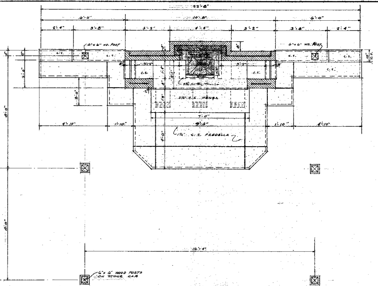
PLAN ABOVE MENSA SCALE: 1/8"=1'-0"
