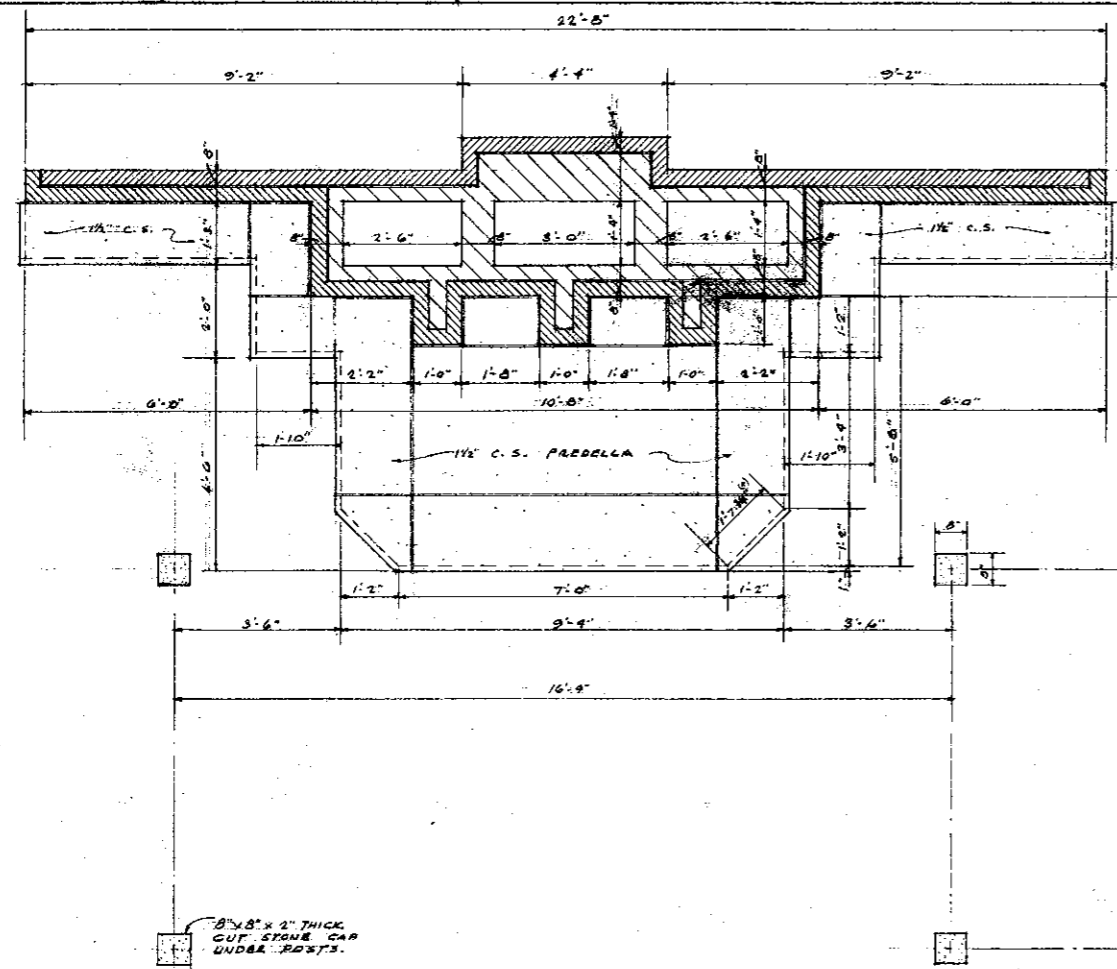
PLAN BELOW MENSA SCALE: 1/8"=1'-0"
